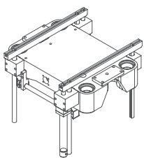
Core ejector / 吊模裝置
