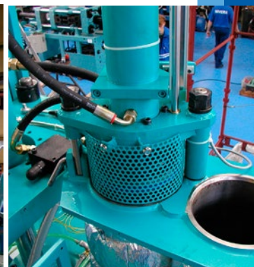
Vstříkovací válec se snímačem dráhy
