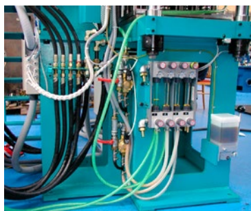
Chladič systému formy stroje
